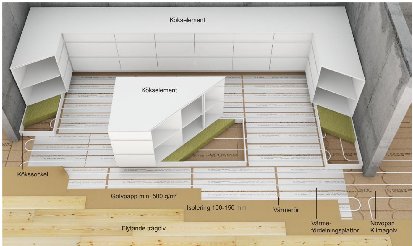
Figur 1 Placeringen av köksskåp markeras på betongplattan, så att vändspår kan utföras under socklarna.
