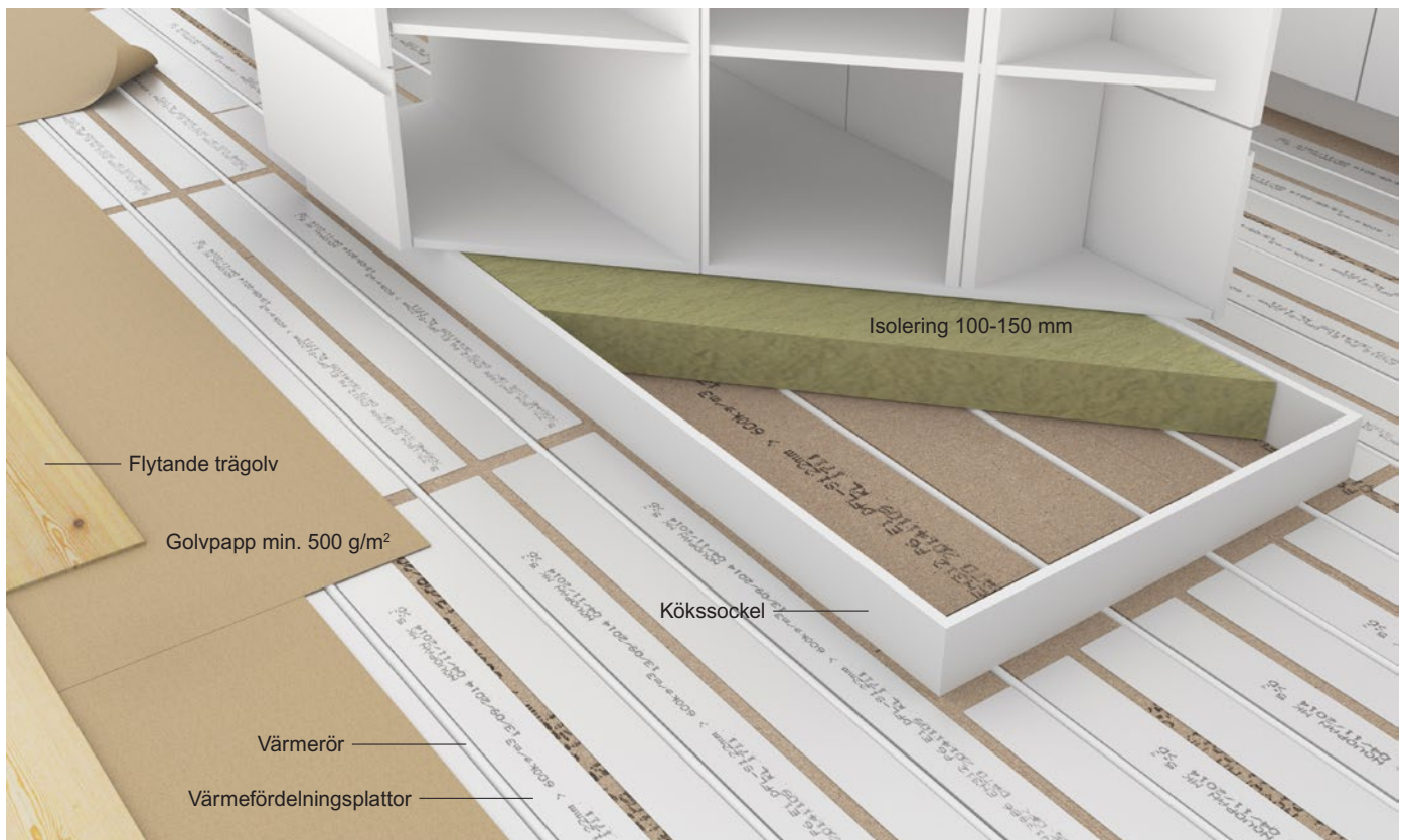
Figur 2 Socklar under köksskåp skall isoleras med 100-150 mm mineralull för att undvika uppvärmning av sockelutrymmet.
